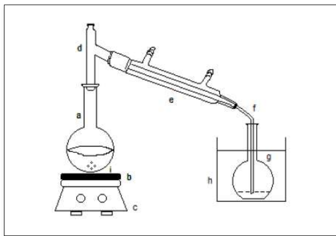
Figura 2-3: Aparato de destilación
