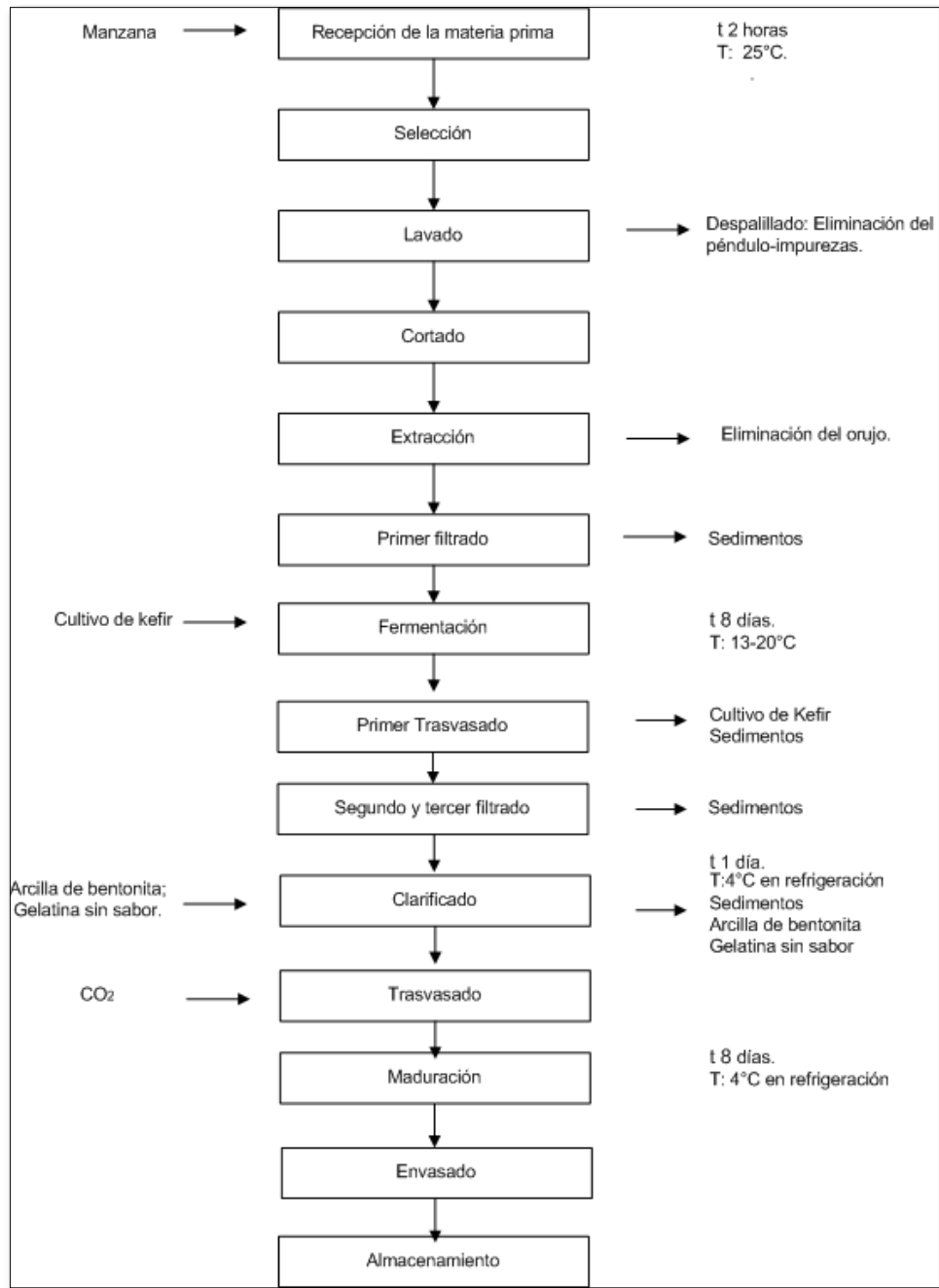
Ilustración 1-3: Diagrama de procesos de la bebida fermentada a base de manzana Delicia Dorada ( Malus Domestica ) con la utilización del cultivo Kefir ( Kluyveromyces Marxianus ). Realizado por: Evelin Chicaiza, 2018
