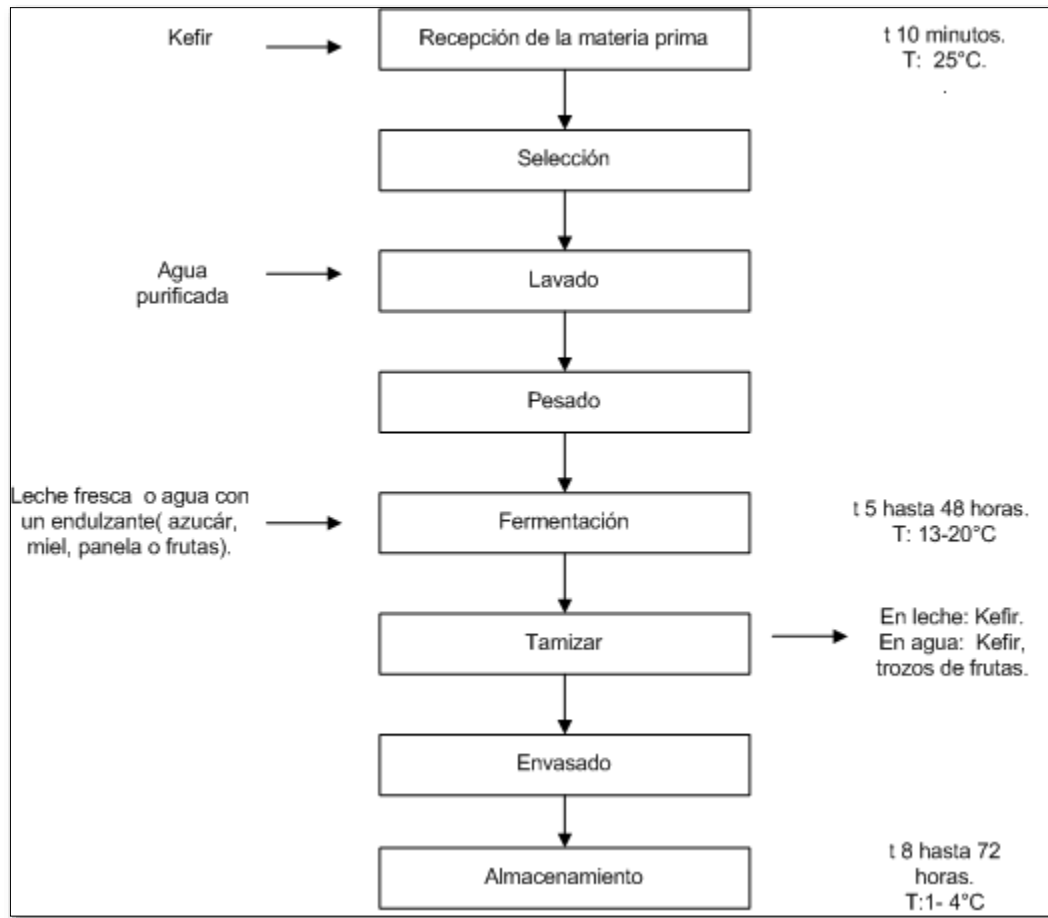
Ilustración 2-2: Diagrama de procesos de elaboración tradicional del cultivo de Kefir ( Kluyveromyces Marxianus )
