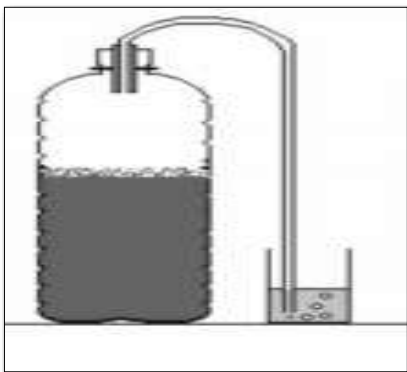
Figura 1-3: Sistema de fermentación
