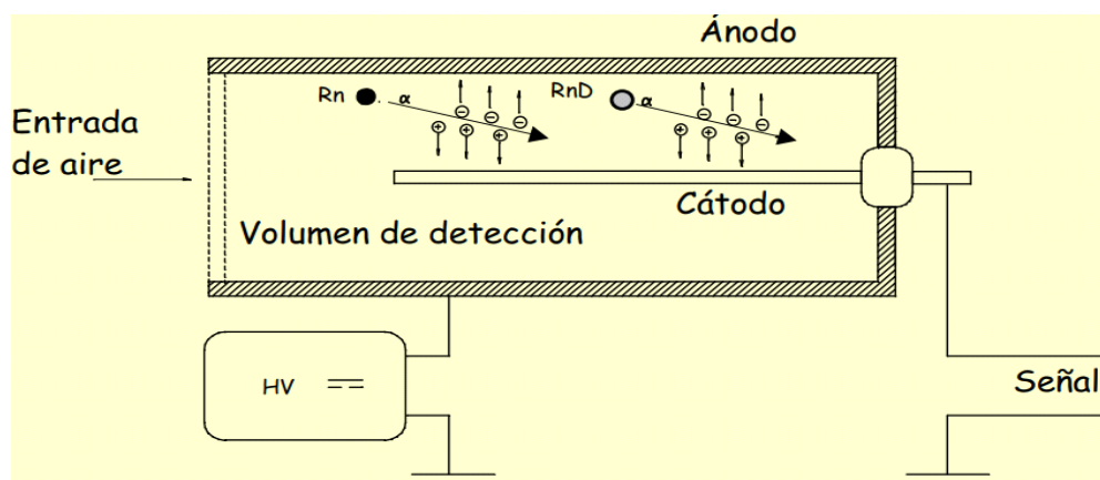
Figura 7-1: Esquema de la cámara de ionización para medición del radón.
